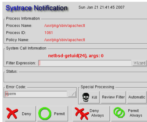
Abbildung 1: Xsysrace bittet den Benutzer um eine Entscheidung
